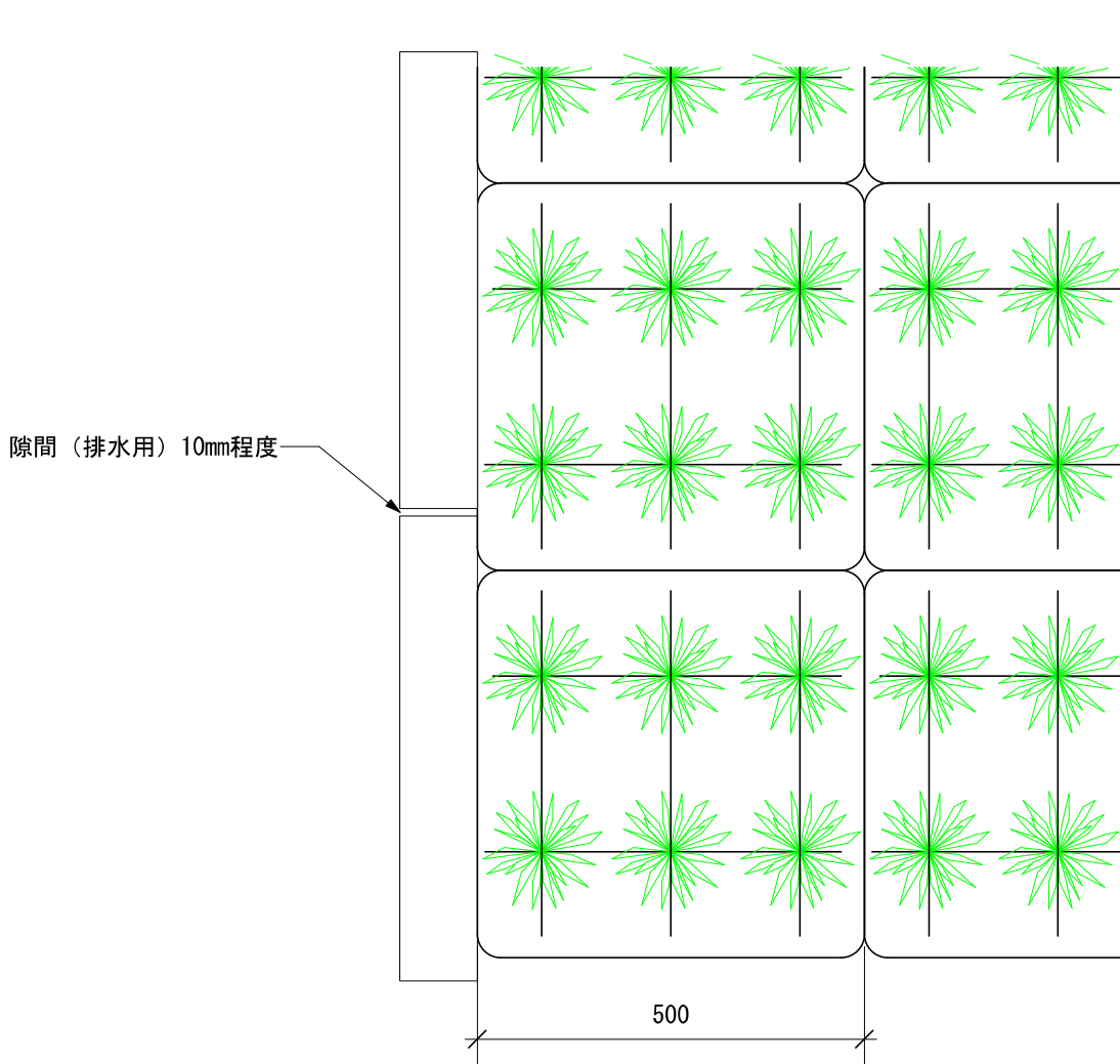
屋上緑化断面図 FTM-NRK
